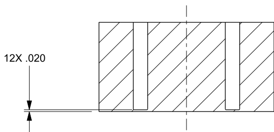
SECCION A-A
