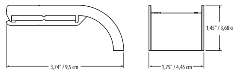
Enrutador compatible con el radio de curvatura
