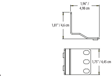
Soporte de montaje
