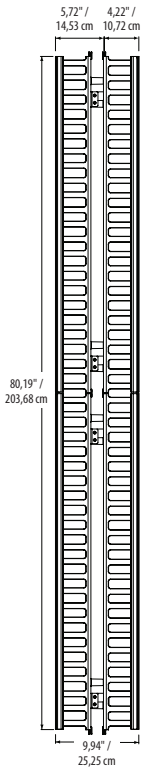
Conducto ranurado vertical (frontal y trasero)
